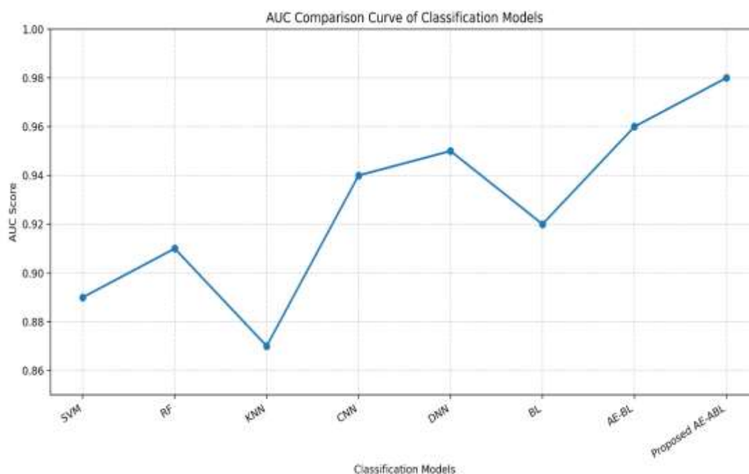
Fig 7. AUC comparison
